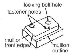
Optional Shim Block
